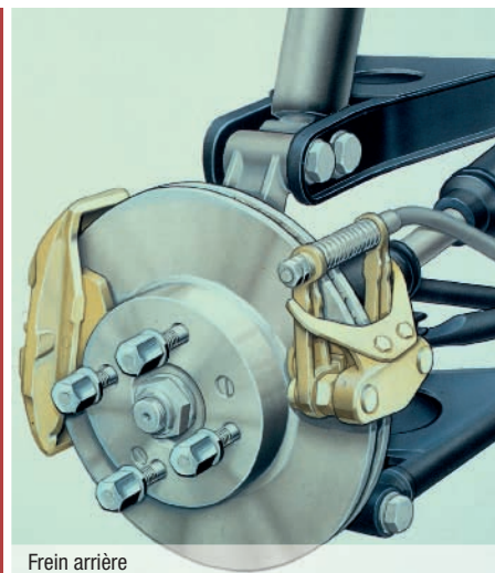
Frein arrière
